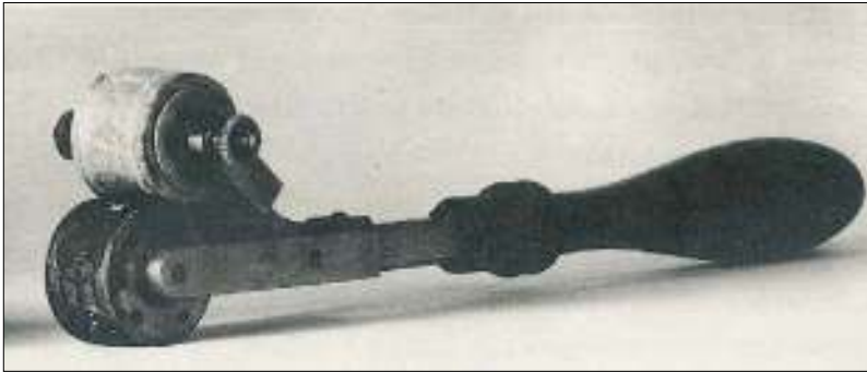
Afb. 1: Drukwerkrolstempel met onderop het rollende stempel; daarboven de inktrol
