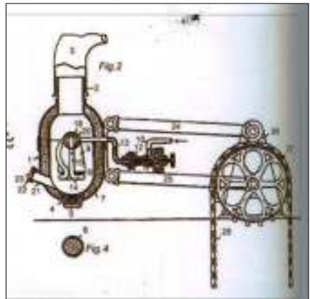
De Vulcanus heetstempelmachine in het echt en schematisch op werktekening
